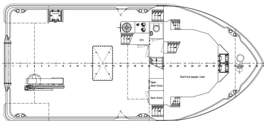
MAINDECK
